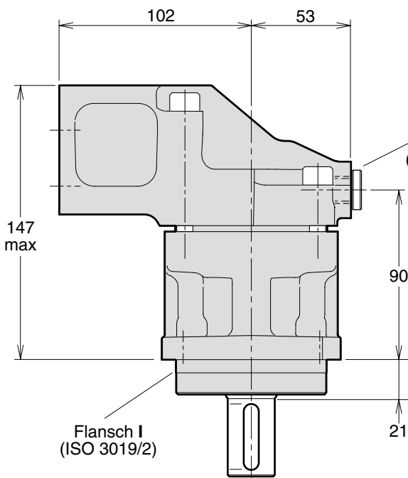
Befestigungsflansch I (ISO 3019/2)
