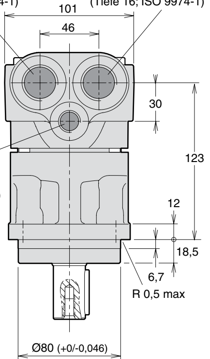
Drainageanschl. C M16x1,5 (Tiefe 12; ISO 9974-1)
