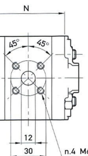
ALBERO FRESATO FORATURA QUADRATO
