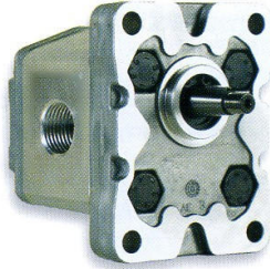
ALBERO CONICO FORATURA GAS 3/8
