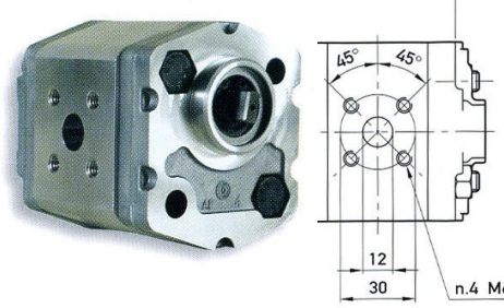
ALBERO FRESATO FORATURA QUADRATO
