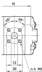
ALBERO FRESATO FORATURA QUADRATO
