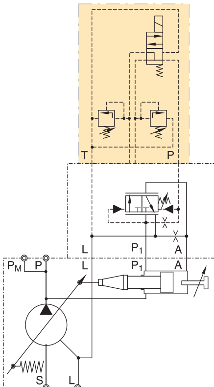
Schaltplan PVAC2P*
