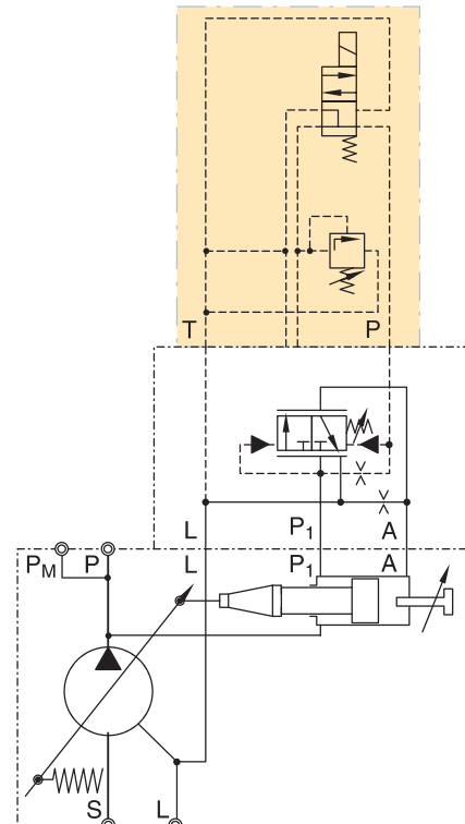
Schaltplan PVAC1E*
