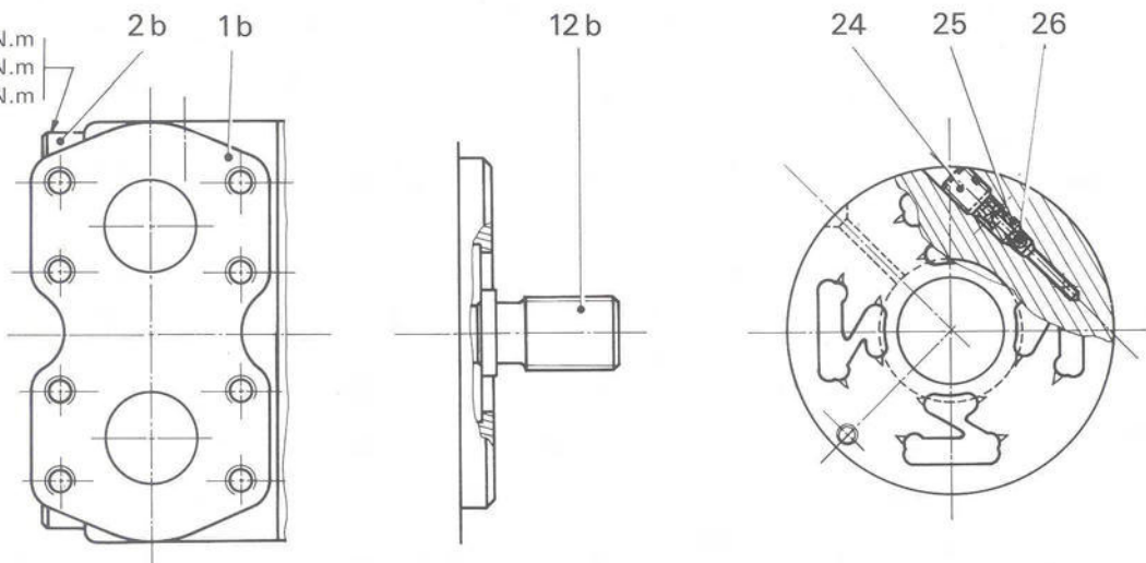
Detail M1C1 rear and side porting - Detail M1C1 axiale und seitliche Anschlüsse - Détail M1C1 orifices arrière et de côtés.
