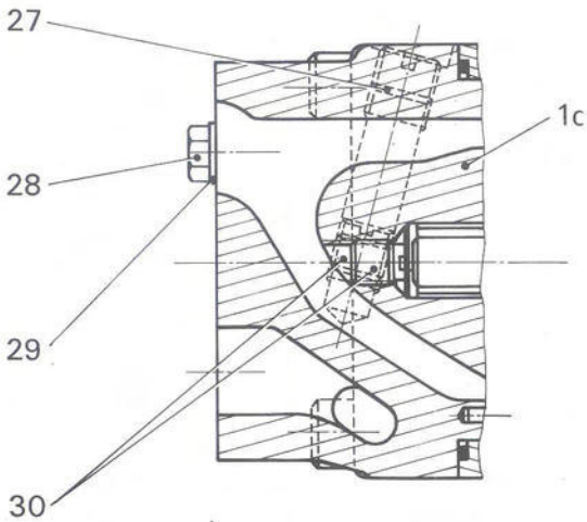
Detail M1C1 rear and side porting - Detail M1C1 axiale und seitliche Anschlüsse - Détail M1C1 orifices arrière et de côtés.
