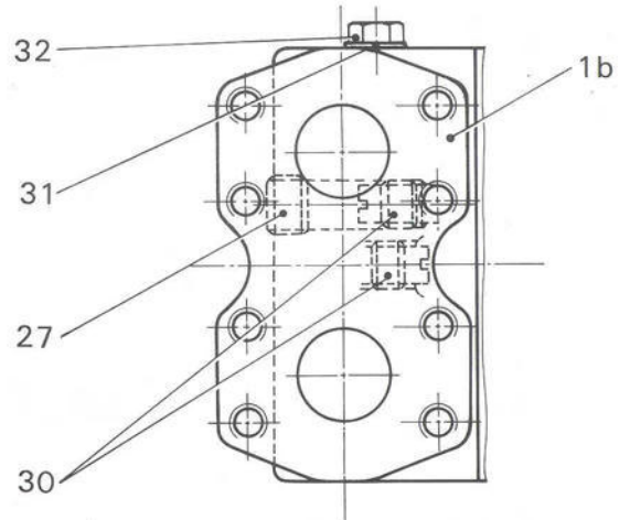
Detail M1C1 rear and side porting - Detail M1C1 axiale und seitliche Anschlüsse - Détail M1C1 orifices arrière et de côtés.
