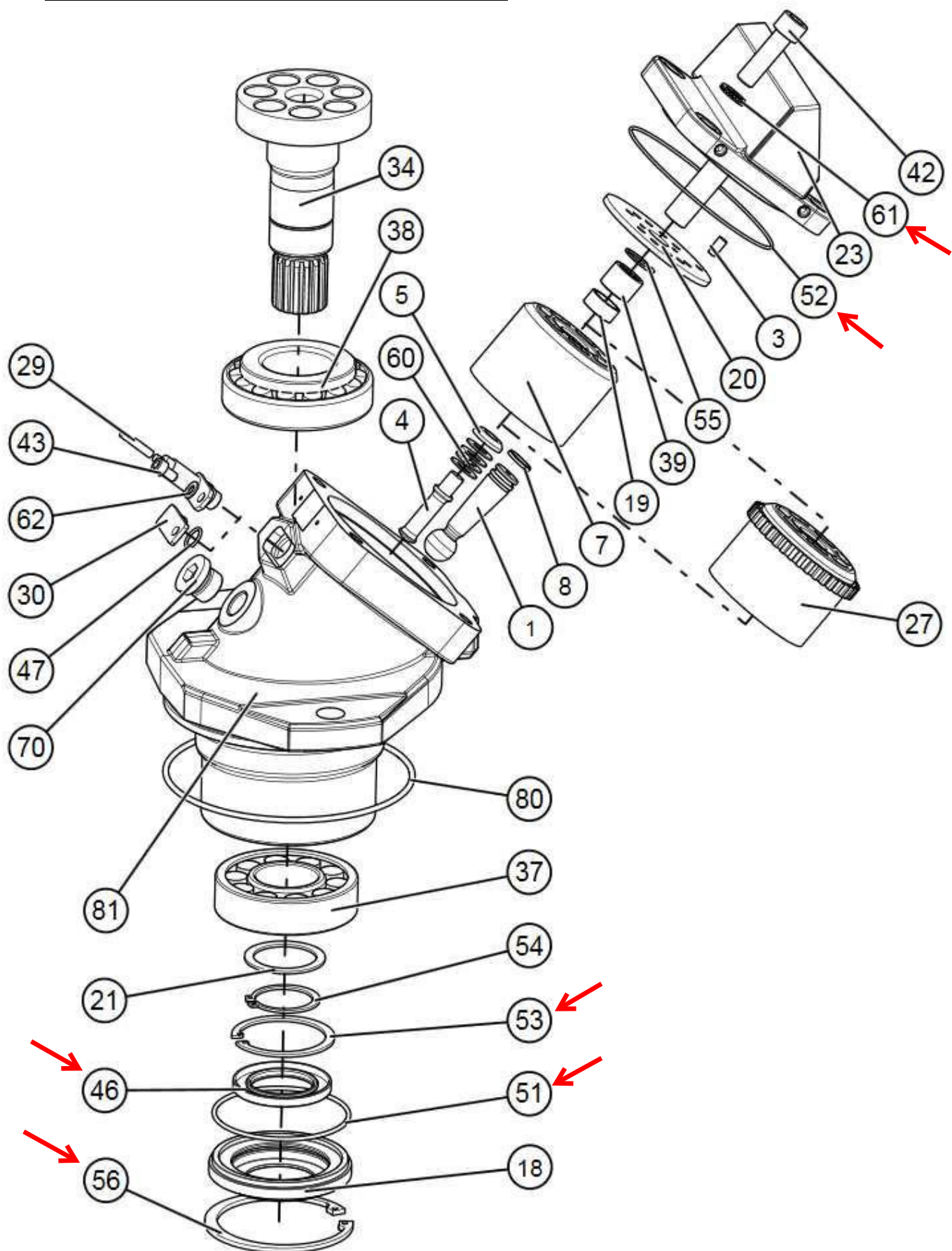
Vue éclatée série MSI / Exploded view MSI series :
