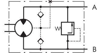
EPMMD mit eingebauten Druckbegrenzungsventilen A ↔ B, Δp = 100 bar(50 bar)
