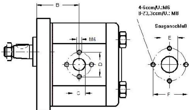
Pumpe mit Flanschanschlüssen Darstellung: rechtsdrehend
