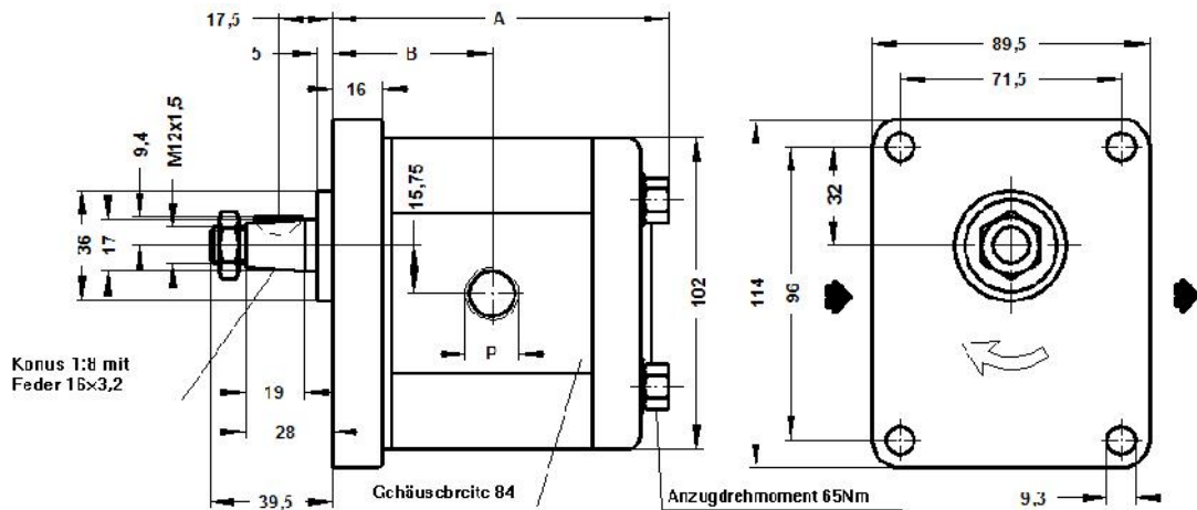
Pumpe mit Gewindeanschlüssen Darstellung: rechtsdrehend
