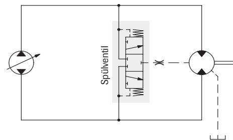
Vereinfachter Schaltplan
